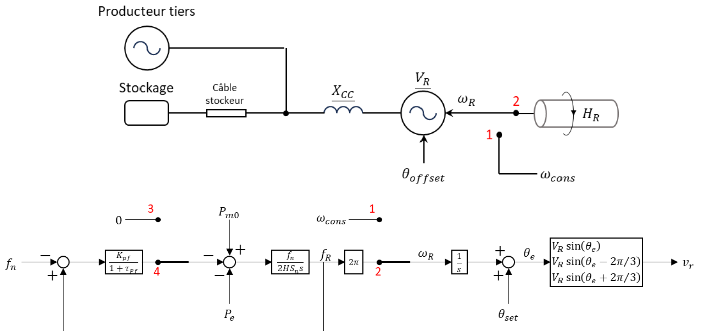
Figure 18 : modèle réseau pour la fiche 3
