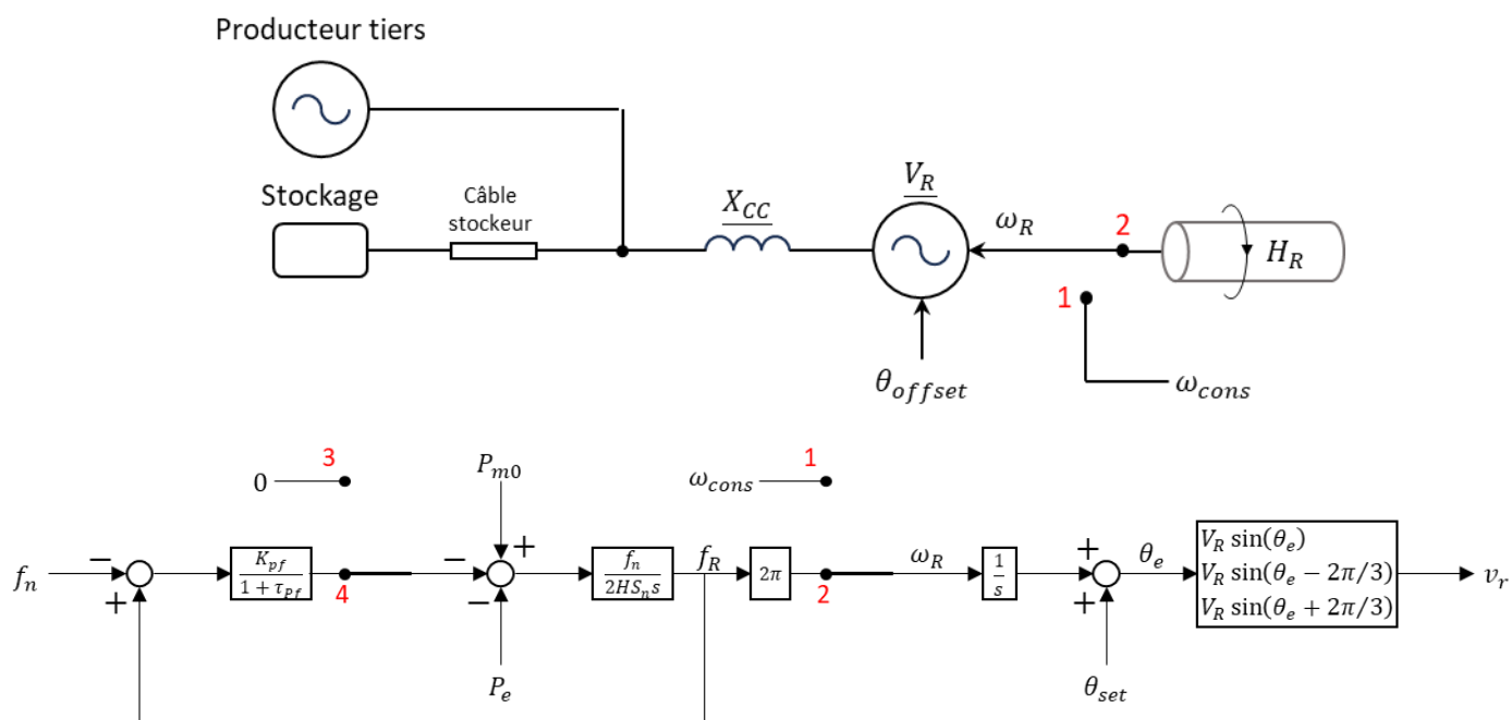
Figure 17 : modèle réseau pour la fiche 2
